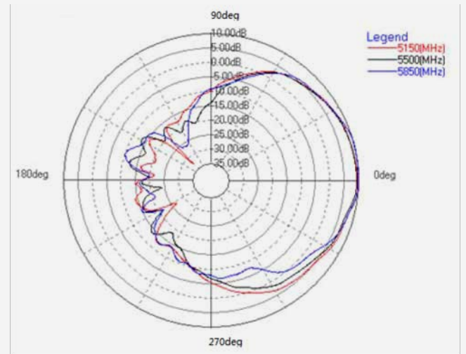
5G (PHI=90)
