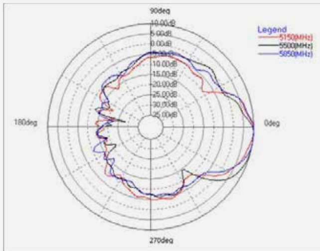
5G (PHI=0)
